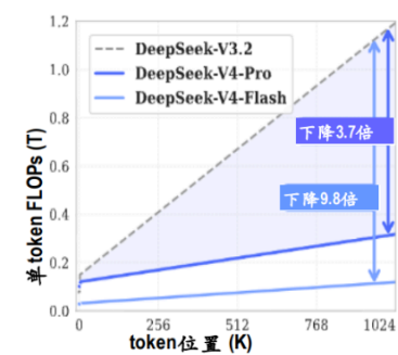
图 2：DeepSeek V4 与 V3.2 的推理 FLOPS 对比
