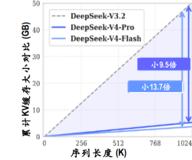
图 3：DeepSeek V4 与 V3.2 的累计 KV 缓存大小对比
